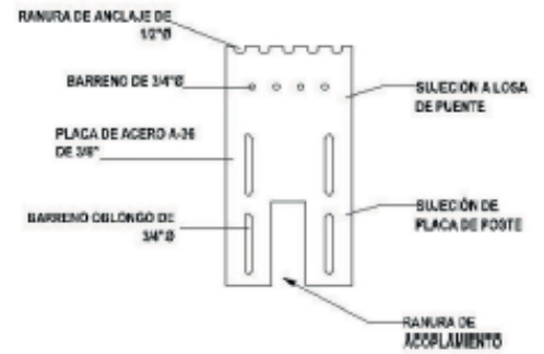
PLACA BASE
