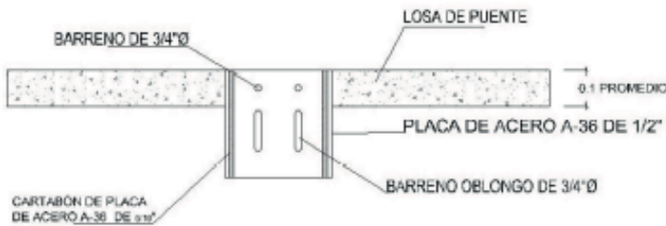
VISTA FRONTAL PLACA BASE
