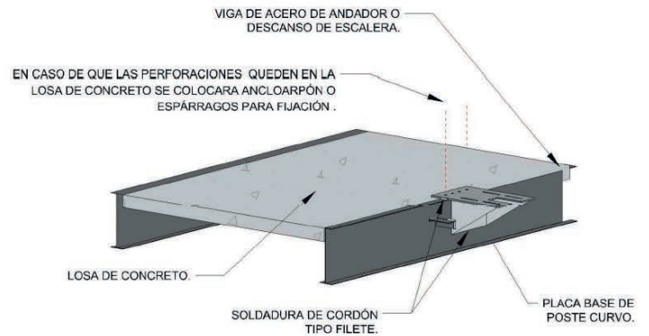
FIJACIÓN MIXTA EN LOSA DE PUENTE
