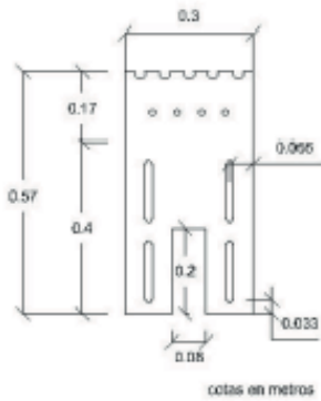
DIMENSIONES PLACA BASE
