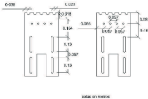
DIMENSIONES DE BARRENOS
