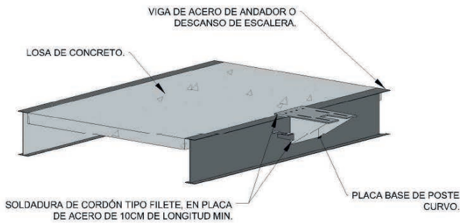
FIJACIÓN EN LOSA DE PUENTE
